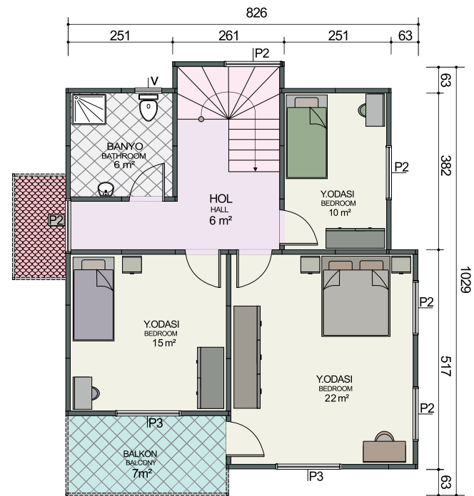
1. Kat Planı / First Floor Plan 68 m 2 + 7 m 2 = 75 m 2
