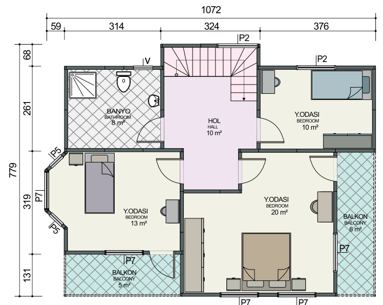
1. Kat Planı / First Floor Plan 66 m 2 + 11 m 2 = 77 m 2
