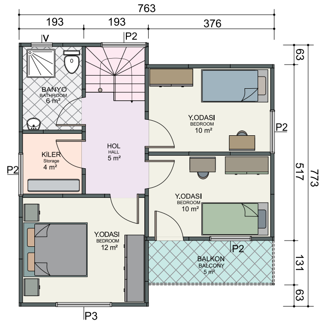
1. Kat Planı / First Floor Plan 49 m 2 + 5 m 2 = 54 m 2
