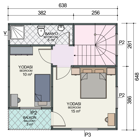
1. Kat Planı / First Floor Plan 38 m 2 + 3 m 2 = 41 m 2
