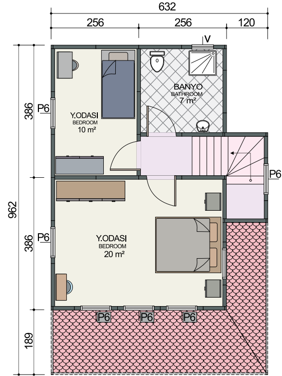
1. Kat Planı / First Floor Plan 42 m 2
