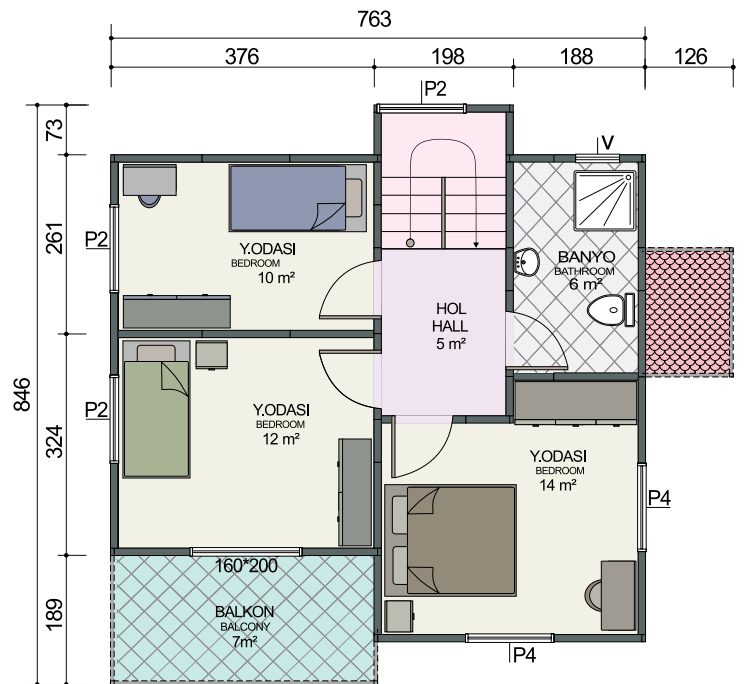
1. Kat Planı / First Floor Plan 51 m 2 + 7 m 2 = 58 m 2
