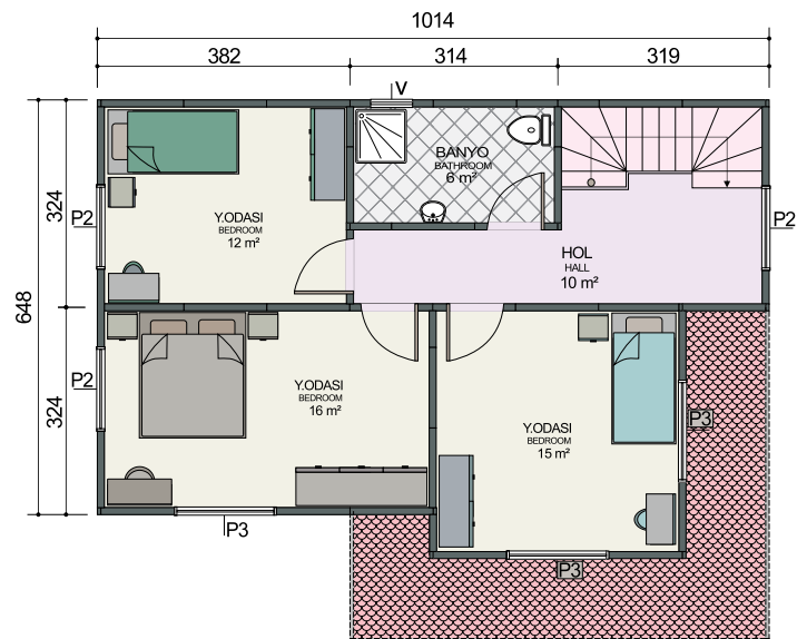
1. Kat Planı / First Floor Plan 64 m 2
