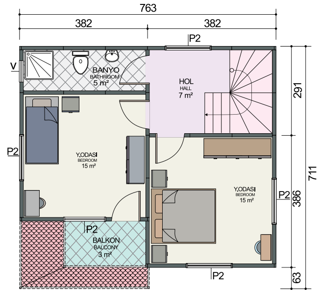
1. Kat Planı / First Floor Plan 45 m 2 + 3 m 2 = 48 m 2
