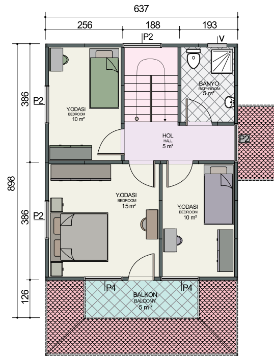
1. Kat Planı / First Floor Plan 49 m 2 + 5 m 2 = 54 m 2
