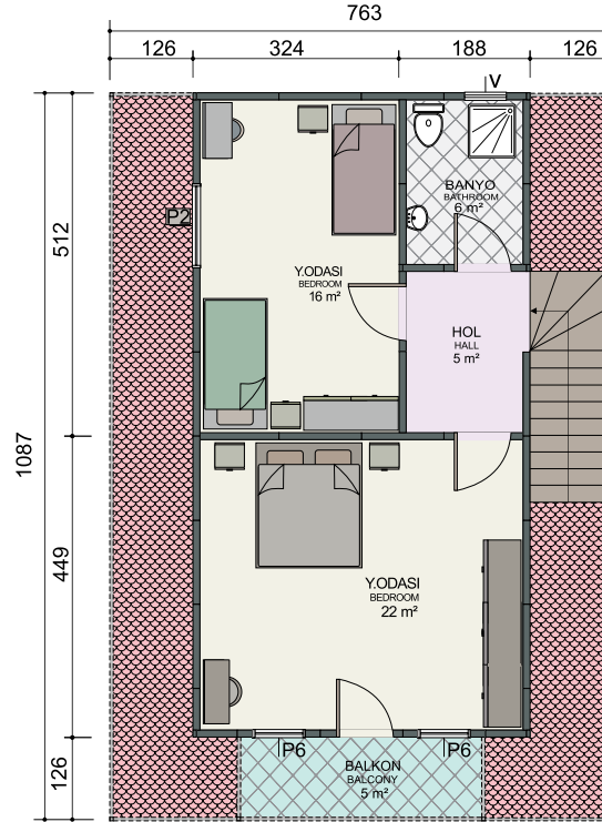
1. Kat Planı / First Floor Plan 50 m 2 + 5 m 2 = 55 m 2
